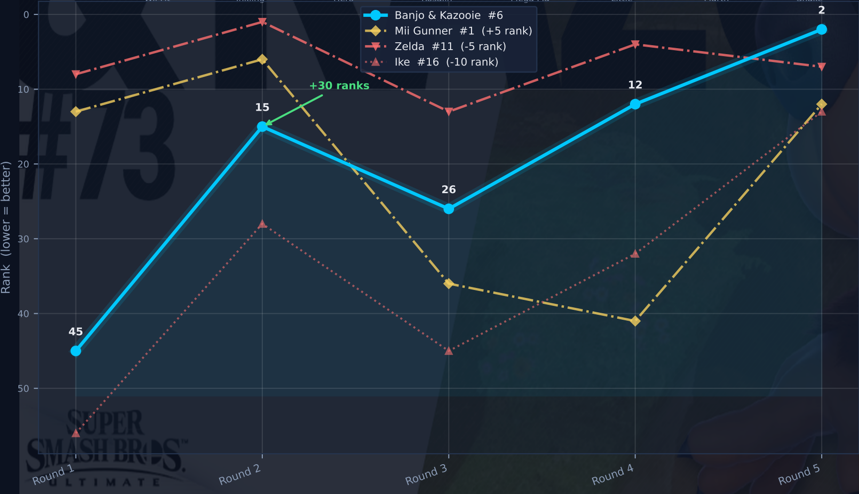
Rank Trajectory
