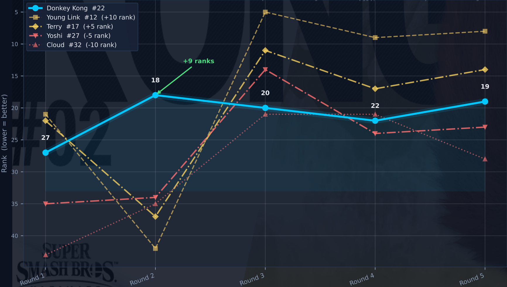
Rank Trajectory
