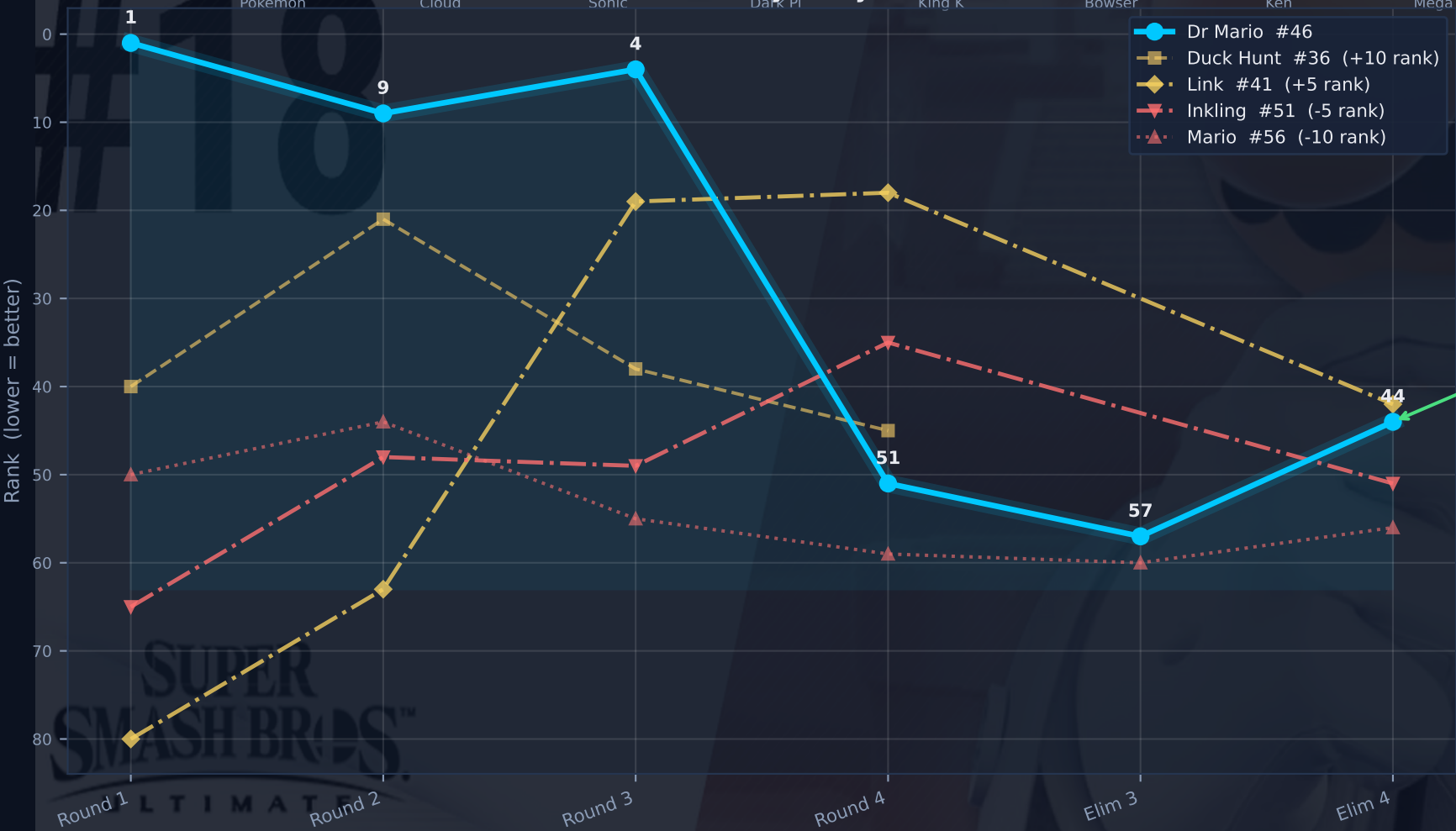
Rank Trajectory
