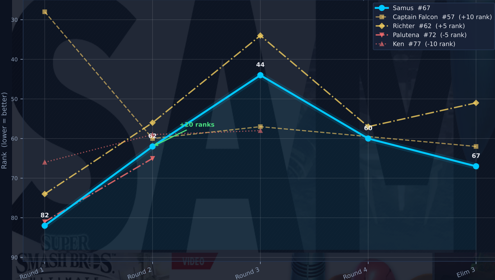
Rank Trajectory
