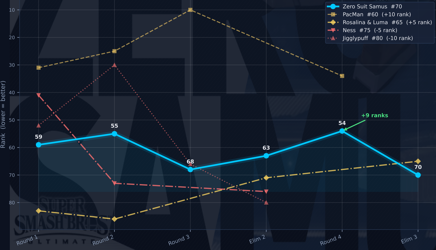
Rank Trajectory
